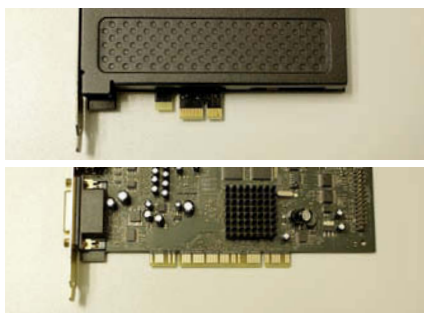
Ein PCI-Express-1x-Anschluss (oben) ist trotz höherer Datenrate deutlich kürzer als die ältere PCI-Variante (unten).
